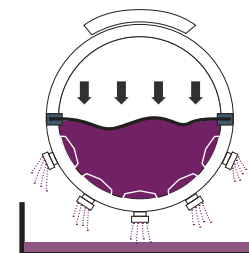
EP2 | Cage fermée volume de cage de pressurage de 15 à 65 hl
