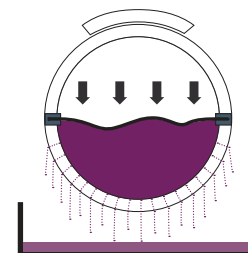
EP1 | Cage ouverte volume de cage de pressurage de 15 à 65 hl
