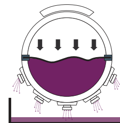
EP3 | Cage mixte volume de cage de pressurage de 15 à 65 hl
